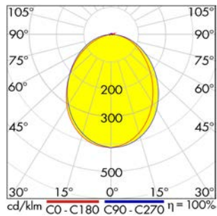
LIHGWA47 (für einen Leuchtenkopf)
