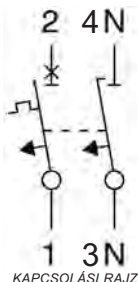
KAPCSOLÁSI RAJZ
