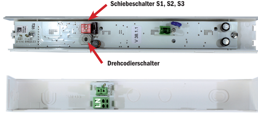
Oberteil mit Klemmen für Durchgangsverdrahtung (max. 2,5mm 2 )
